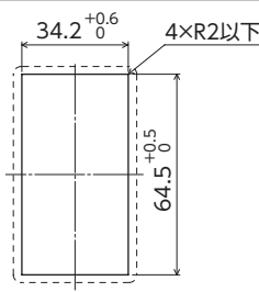
取付穴参考寸法図 [単位: mm]
